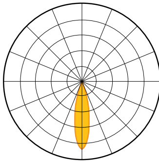
SPOT 29° BEAM ENCASTRÉ FAISCEAU DE 29°
